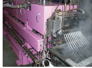
2軸押出機
