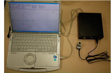
手術中に使用可能な加速度センサーを使用した角度計
