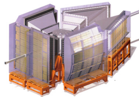
超高分解能中性子回折装置 BL-08
