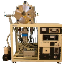
5源スパッタ装置
