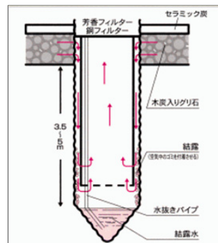
地中熱利用のGEOパワーシステム (ジオパイプ)
