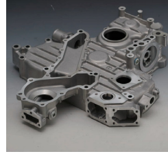
小型ディーゼルエンジン用 ギヤケース
