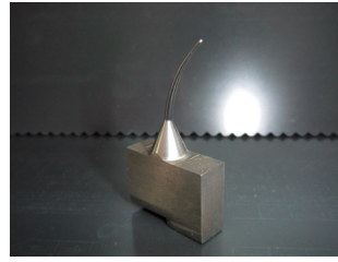
削り出し湾曲コアピン(医療部品)
