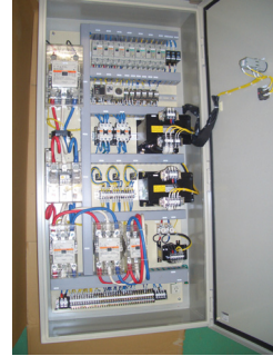
制御盤
