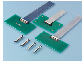
極細同軸ケーブル用コネクタ (SSL/USL/USLSシリーズ)
