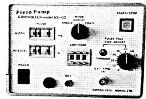
コントローラー NS-02D
