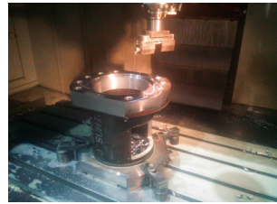
溶接構造品精密加工 各部幾何公差(直角、同芯) 0.02
