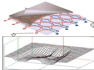
電磁誘導方式圧力分布センサー
