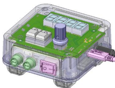
ペットコントローラ
