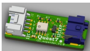
I2Cバス延長基板
